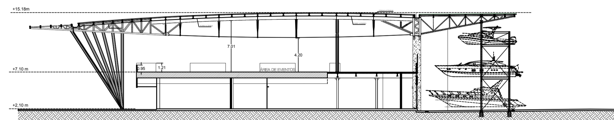
CORTE TRANSVERSAL ESC.: 1/750
